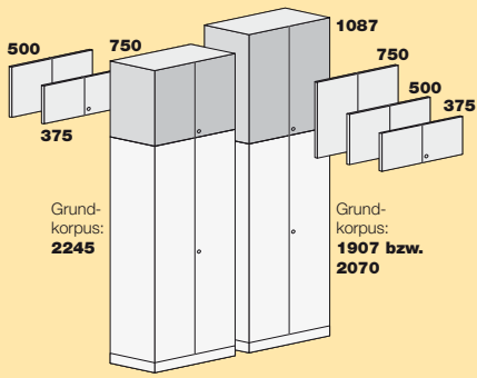
Elementhöhen (Schranksätze)
