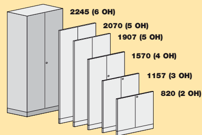
Elementhöhen
