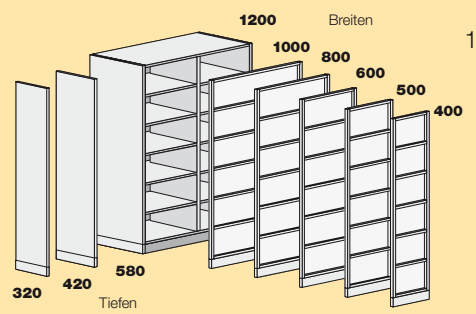
Elementtiefen und -breiten für Regale
