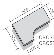
CP.QSTP22L CP.QSTP22R
