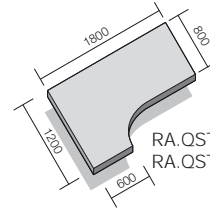
RA.QSTP22L RA.QSTP22R
