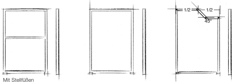
Mit Stellfüßen
